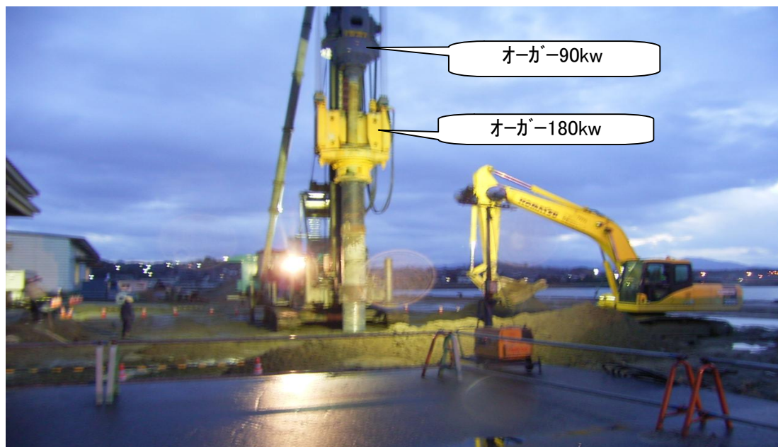
《施工状況 全景》
